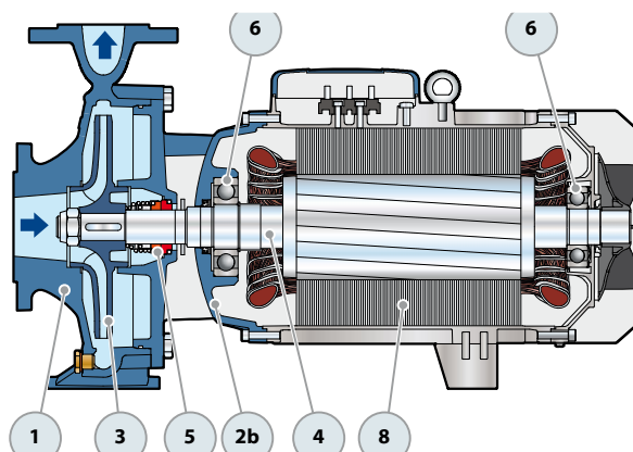
Trójfazowa wersja
