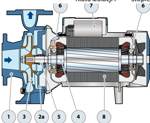
Jednofazowa wersja
